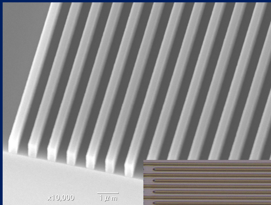
0.5ミクロン L&S: 上(SEM)、右(光学顕微鏡)
