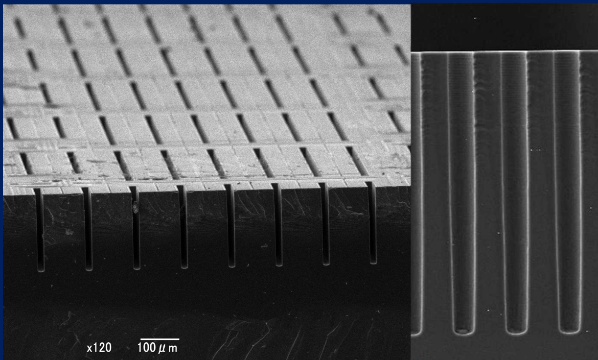
200ミクロン 深掘り
