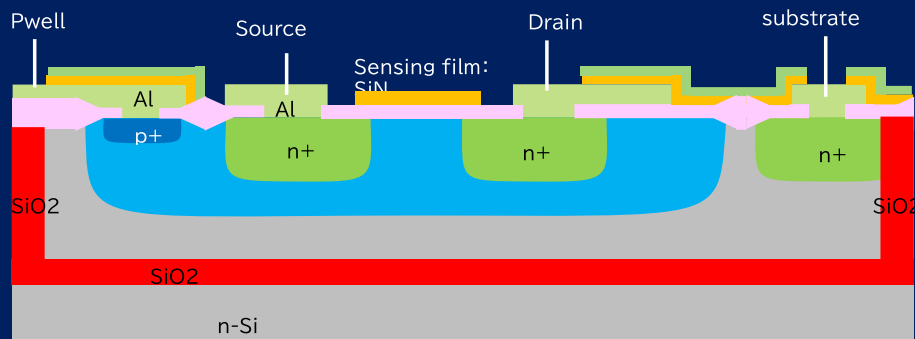
図1:絶縁体で覆われたIS-FET
