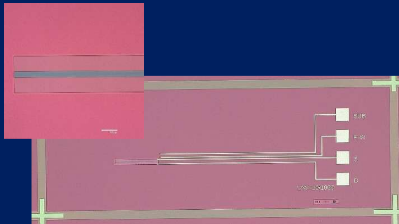
図2:S-FETチップ写真
