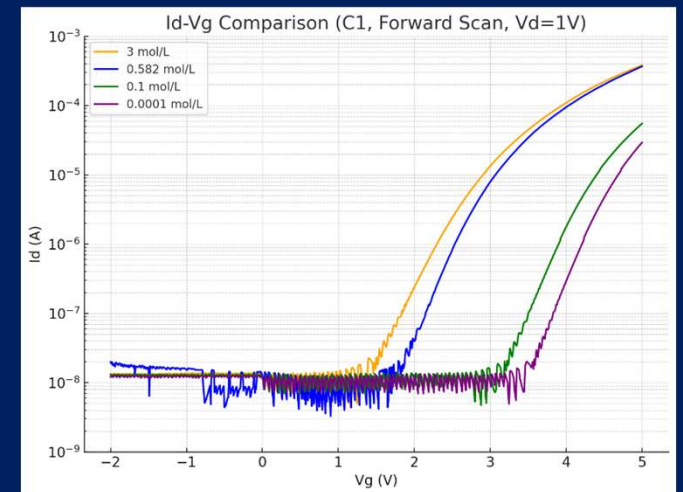
図3:塩水中でのセンサー特性
